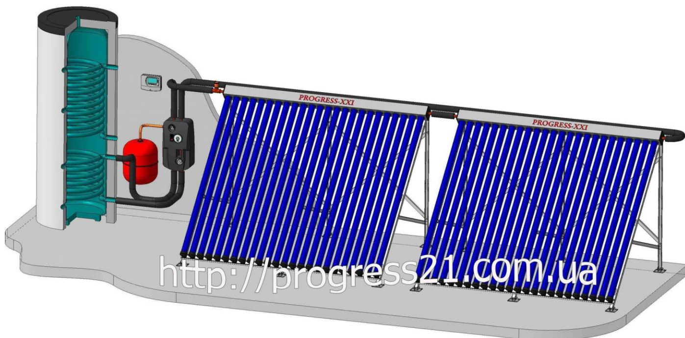
Принципиальная схема гелиосистемы
